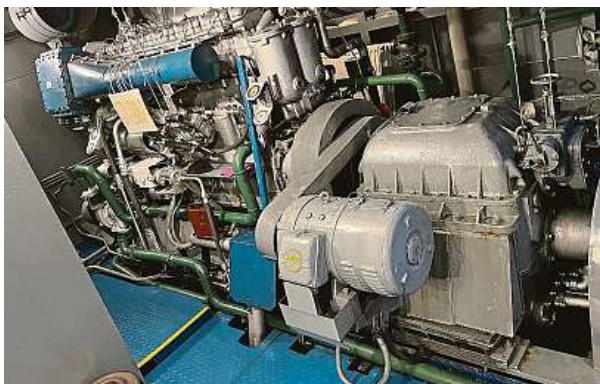
Tlačný remorkér Tankovačka pohání dvojice motorů ČKD 6L 150. Stejně mají i motorové vlaky M 262.
