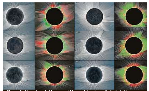
Sluneční koróna během celého cyklu sluneční aktivity
