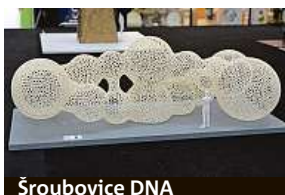
Šroubovice DNA
