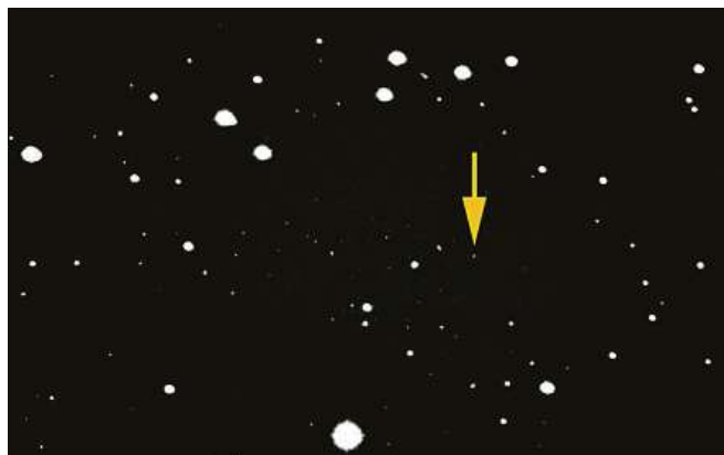
Snímek, na kterém byla objevena planetka (401820) Špilas, vznikl 30. září 1996 pomocí 0,57-m zrcadlového dalekohledu Observatoře Kleť CCD kamerou SBIG ST-8 expozicí 120 sekund. Autoři: Miloš Tichý a Zdeněk Moravec
