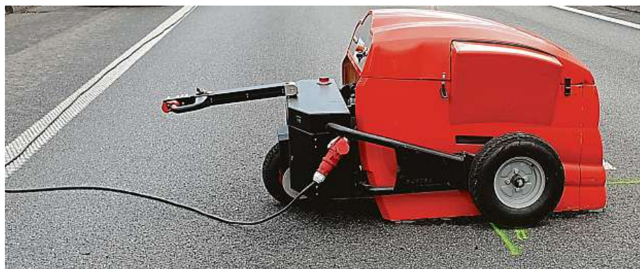
Preventivní údržbu asfaltových vozovek technologií mikrovlnného ohřevu dosud společnost zajišťovala prostřednictvím svého pilotního zařízení FT3. S ním opravila přes tisíc děr a výtluků.
